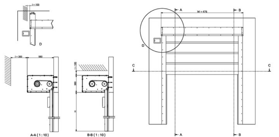
A-A (1:10)
